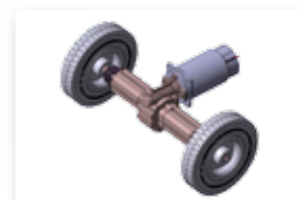
Электрический привод колес с дифференциалом
